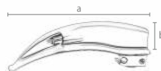
Macintosh Disposable Fiber Optic (F.O.) Laryngoscope Blade.
